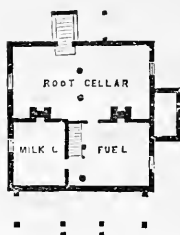
FIG. 117.—CELLAR PLAN.
