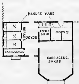
FIG. 51.—PLAN.
