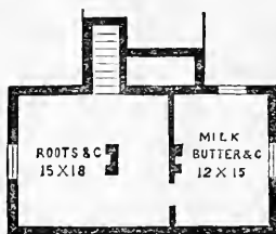
FIG. 16.—CELLAR PLAN.
