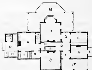
FIG. 121.—GROUND PLAN.
