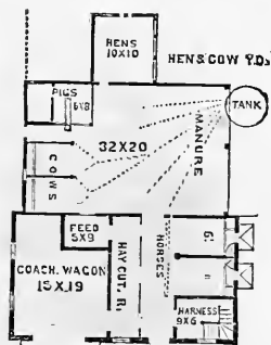
FIG. 67.—GROUND PLAN.
