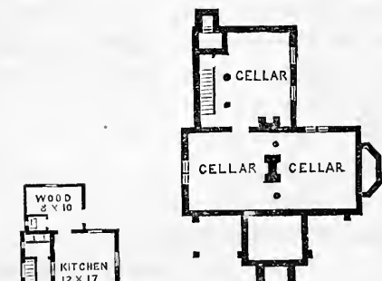
FIG. 73.—CELLAR PLAN.
