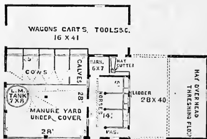
FIG. 138.—PLAN.
