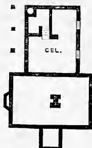
FIG. 154.—CELLAR PLAN.
